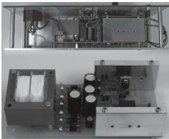
Gleichrichter- und Lastreglerleiste
