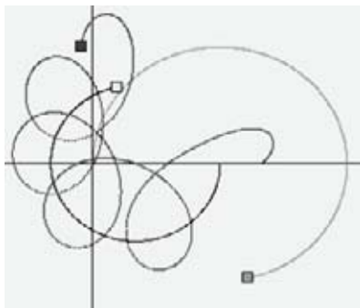
Simulation der Bahn eines Doppelsternsystems
